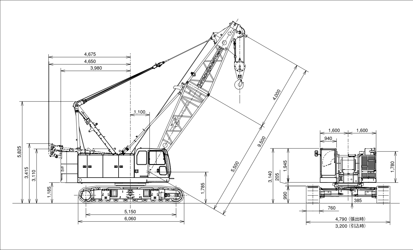
■寸法図
